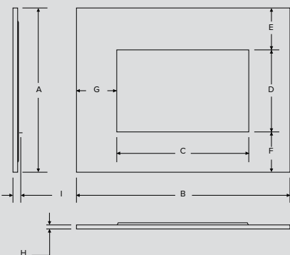
Dimensions contour mural en coin (pouces)
